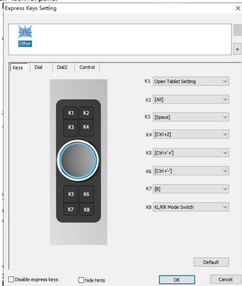
Рис. 3.10. Горячие клавиши
