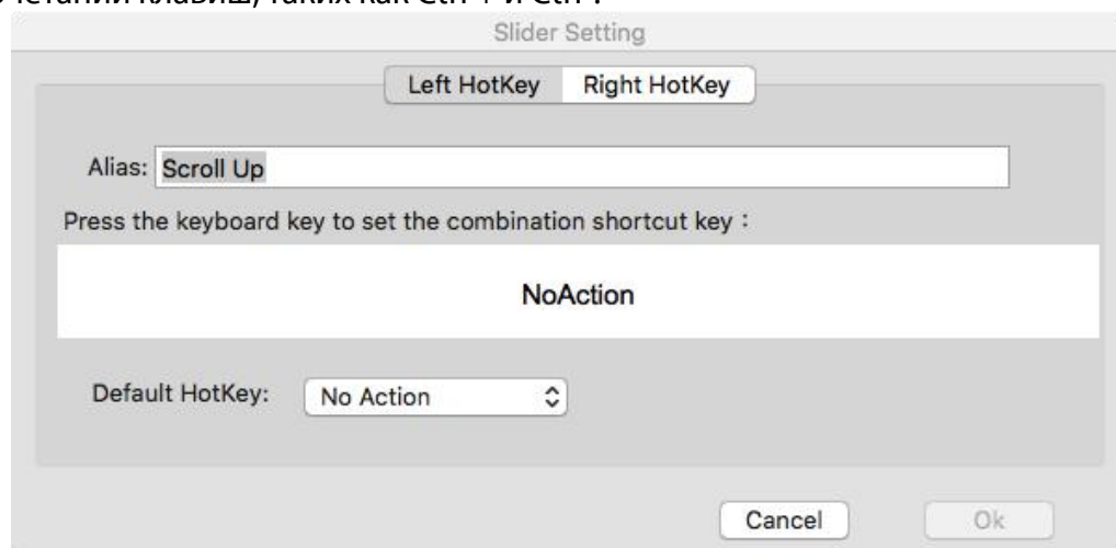
Рис. 3.36. Настройка Slider
