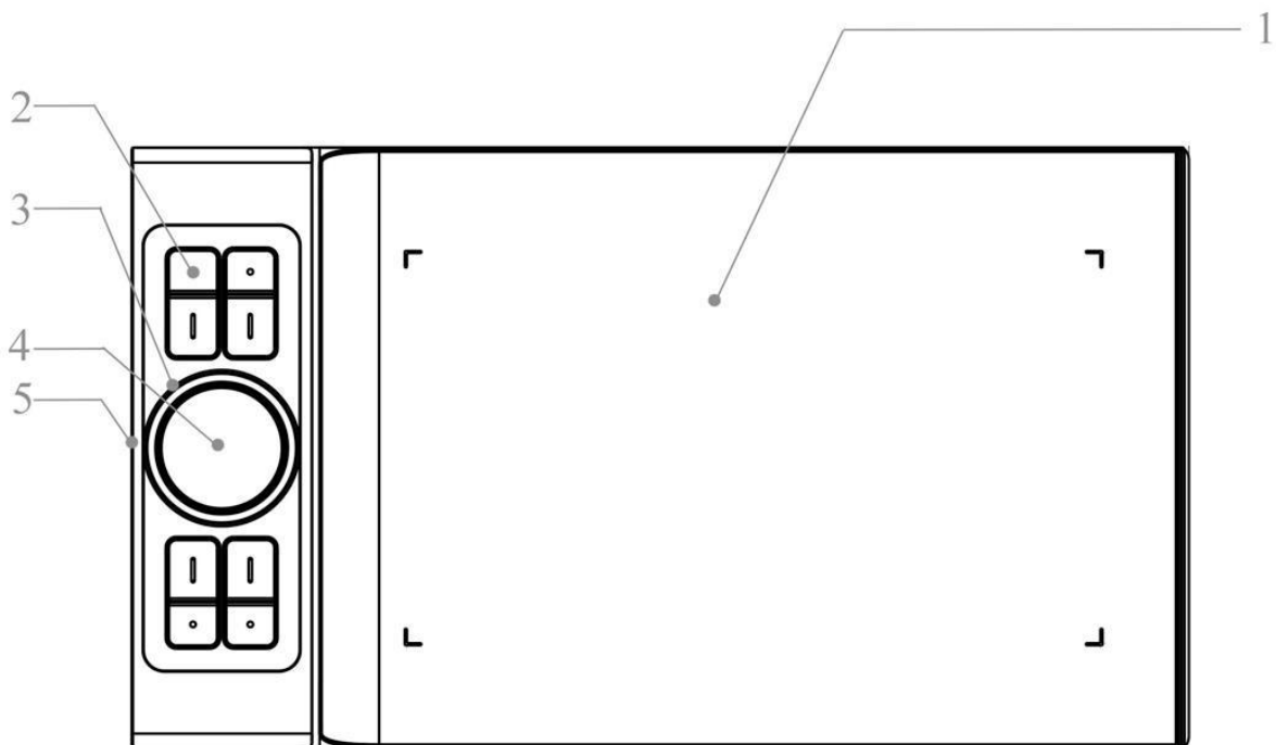
Рис. 1.1. Обзор
