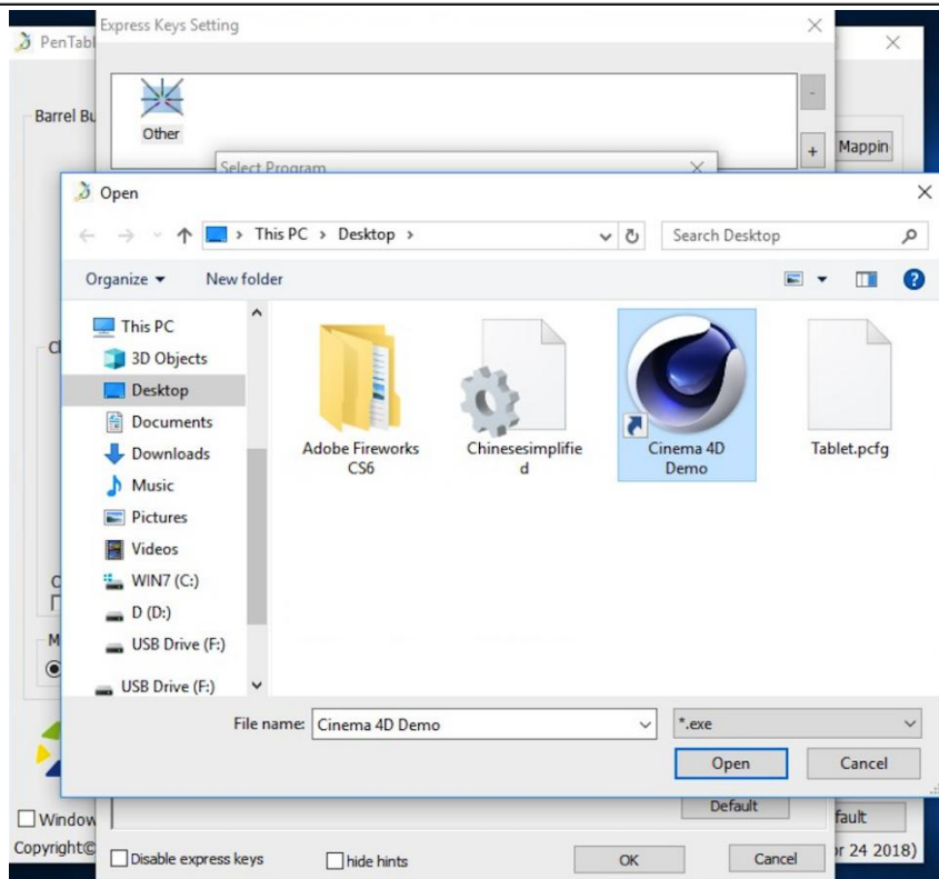
Рис. 3.13. Выбор программы
